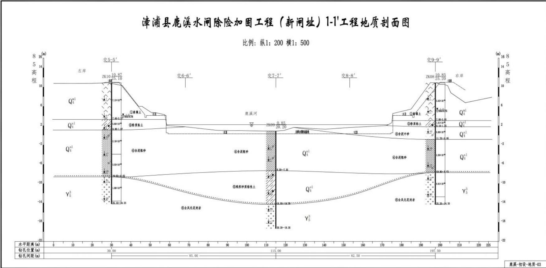
图 4.1-2 典型剖面图 1-1'
