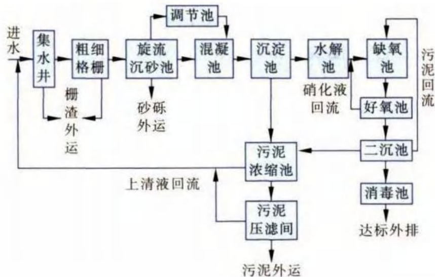
图 6.1-3 大南坂污水处理厂污水处理工艺图
